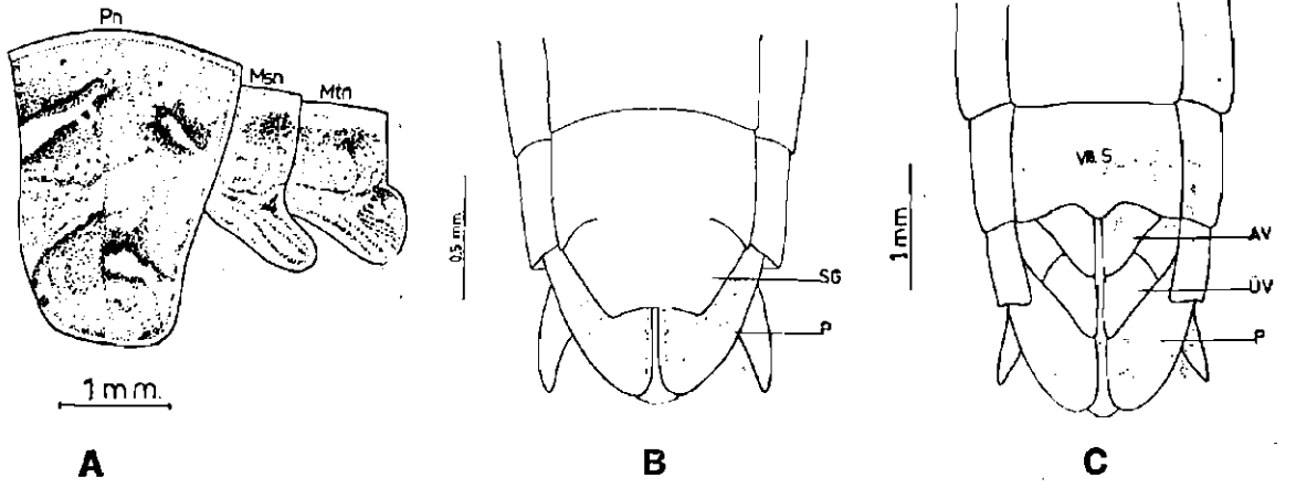
ŞEKİL 6. Üçüncü dönem nimfde - A. Thorax, yandan; B. Erkek abdomeninin sonu; alttan; C. Dişi abdomeninin sonu; alttan görünüşü. AV - Alt ovipositor valv'leri, Msn - Mesonotum, Mtn - Metanotum, Pn - Pronotum, P - Paraproct, SG - Erkekde subgenital plaka, ÜV - Üst ovipositor valv'leri, VIII S - Sekizinci sternit.
